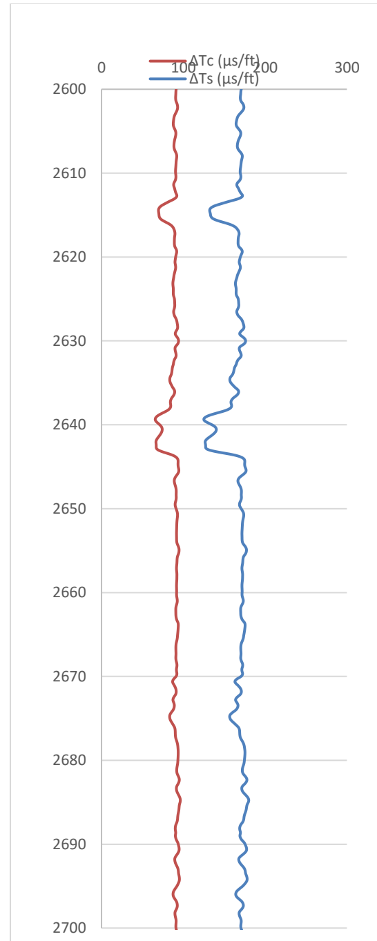
شکل ۱: نمودارهای بدست آمده از چاه در مخزن مورد مطالعه بر حسب عمق
