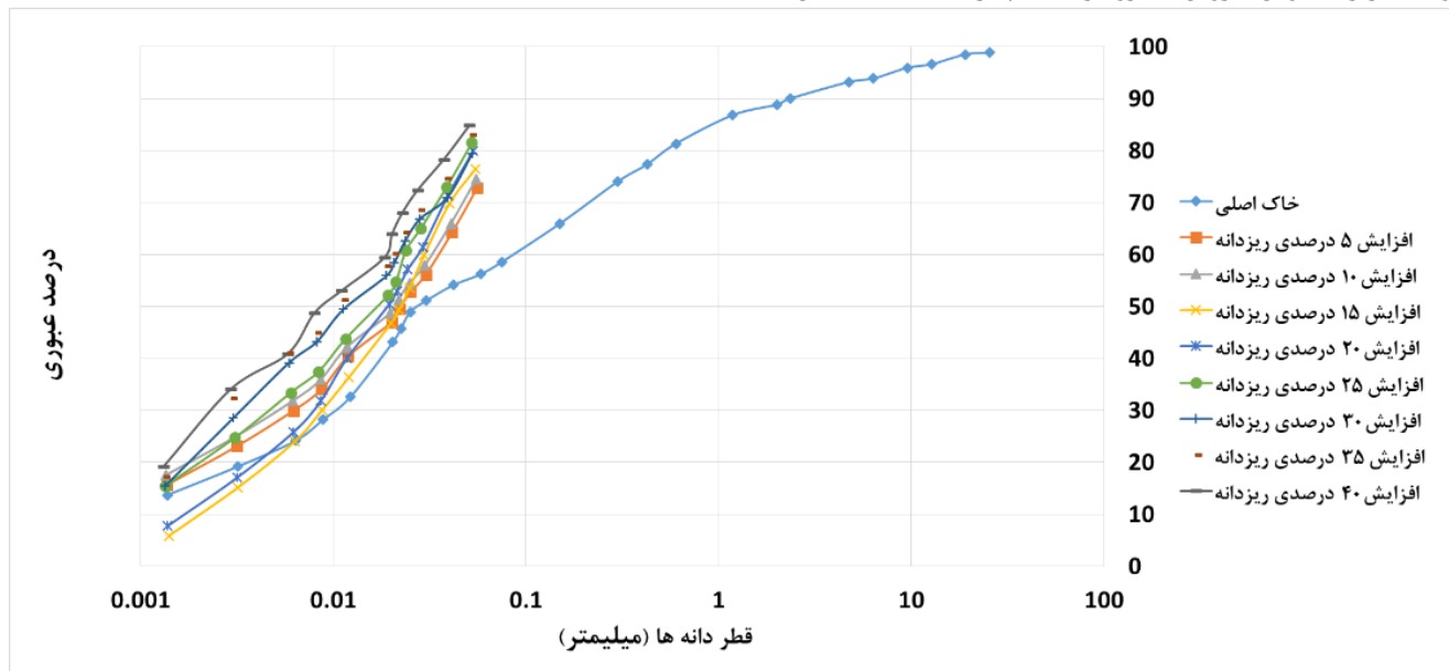
شکل ۷: نمودار دانه‌بندی خاک اصلی مورد آزمایش و خاک‌های با درصد ریزدانه (عبوری از الک شماره ۲۰۰) مختلف.
