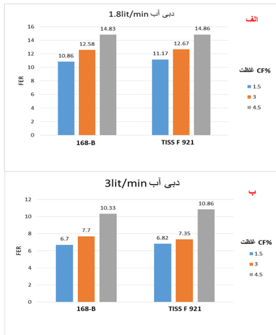
شکل ۱۲: تاثیر غلظت ماده فوم ساز بر میزان FER (الف) دبی آب ۱.۸ lit/min (ب) دبی آب ۳ lit/min.
