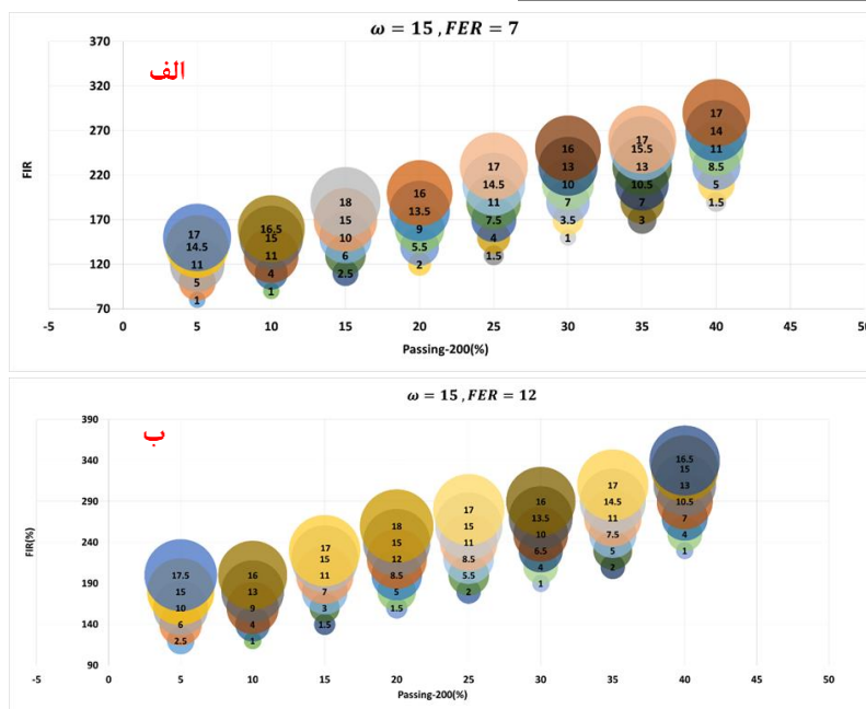
شکل ۱۰: نمودار حبابی برای بررسی رابطه‌ی بین تغییرات درصد ریزدانه خاک (عبوری از الک ۲۰۰) (محور افقی)، مقدار FIR (محور قائم) و میزان افت اسلامپ (اندازه حباب‌ها) برای رطوبت ۱۵ درصد خاک و الف) FER=7 و ب) FER=12.
