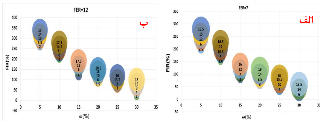
شکل ۸: نمودار حبابی برای بررسی رابطه ی بین تغییرات درصد رطوبت خاک (محور افقی)، مقدار FIR (محور قائم) و میزان افت اسلامپ (اندازه حبابها) برای الف) FER=7 ب) FER=12 .
